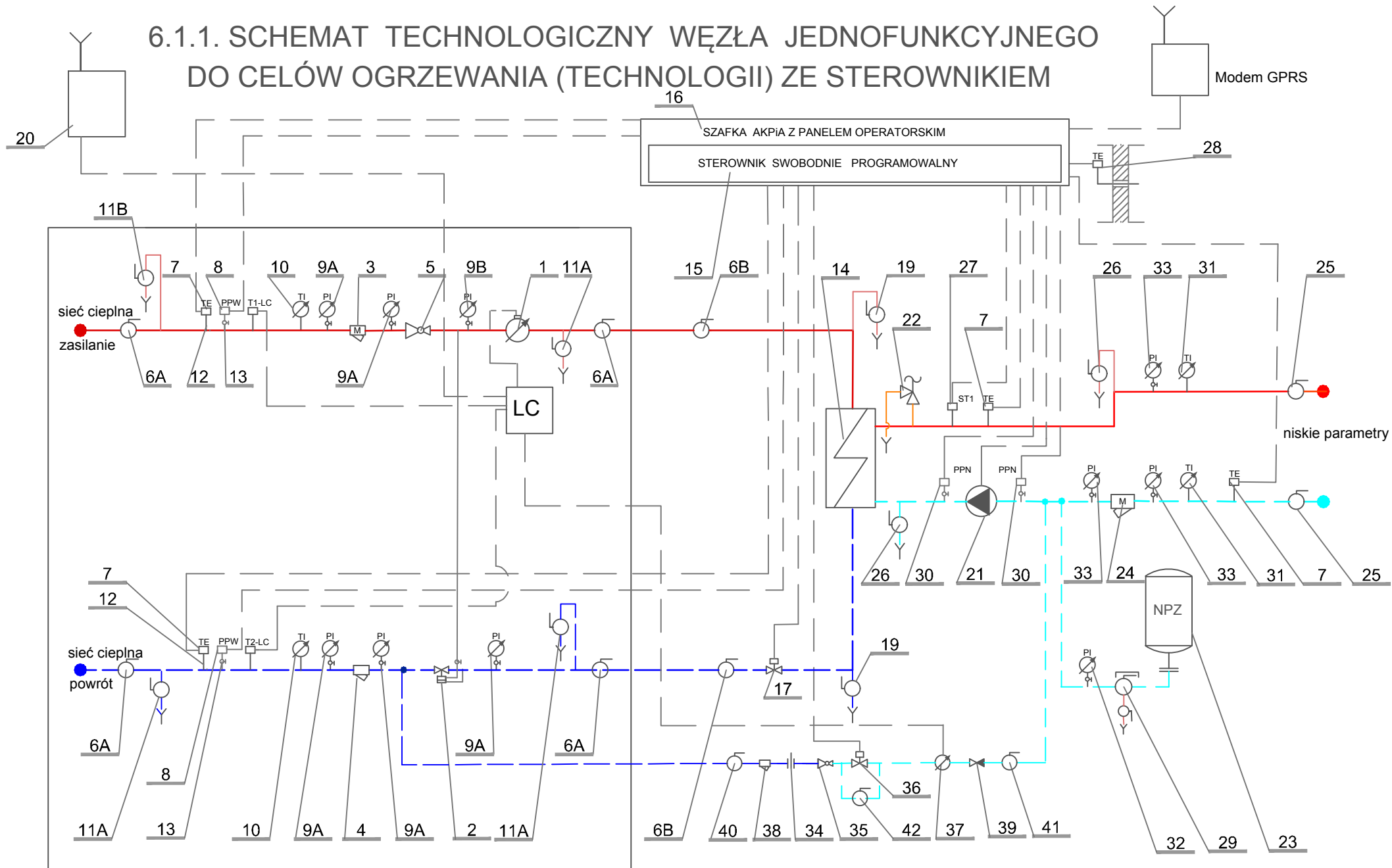
WĘZŁ CIEPLNY C.O. (TECHNOLOGII)
