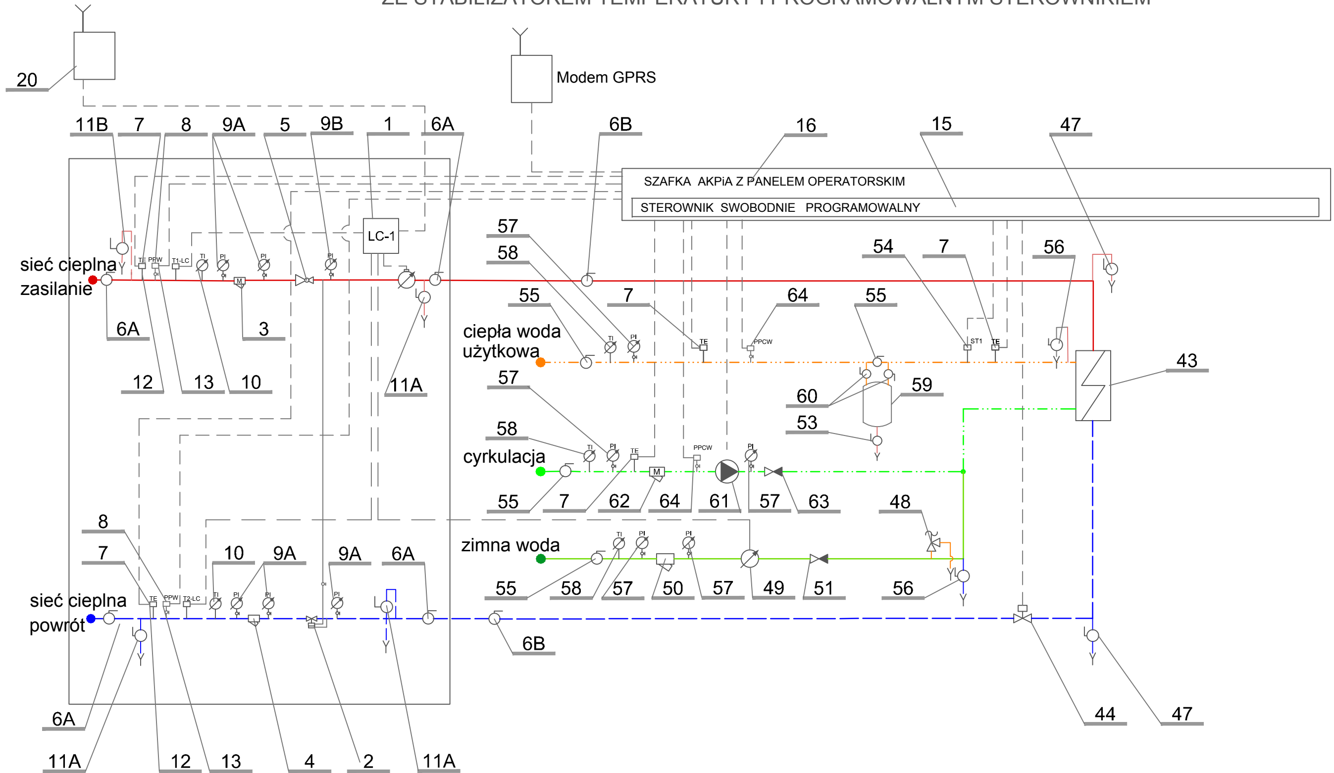
WĘZEŁ CIEPLNY C.W.U. ZE STABILIZATOREM TEMPERATURY
